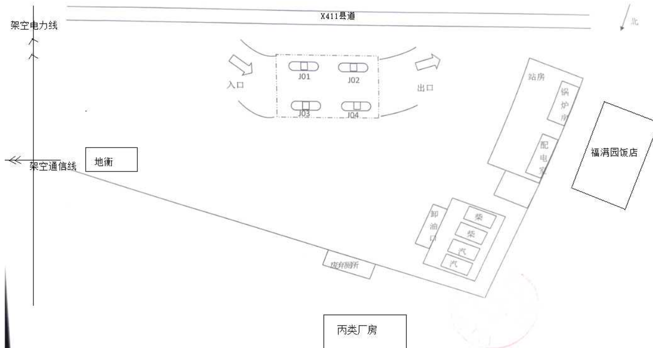
扎赉特旗宝力根花宏达加油站平面布置图
