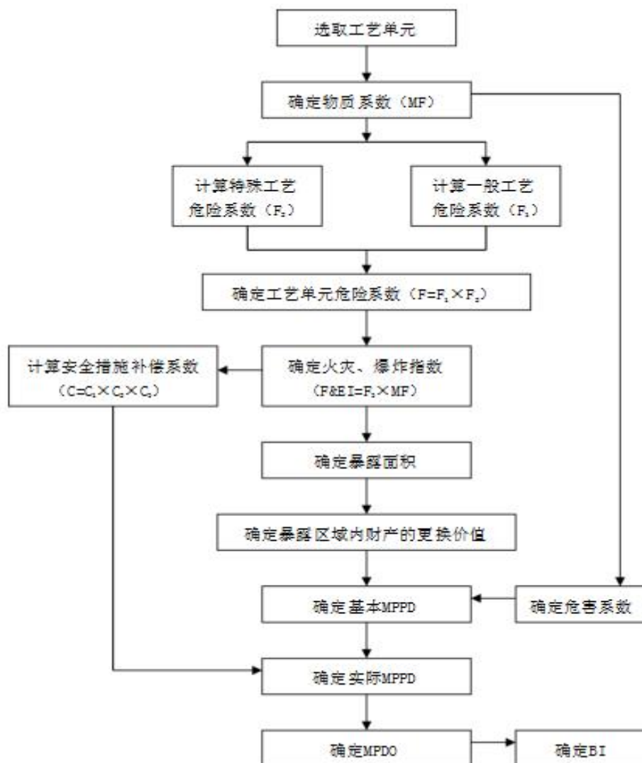
图4.2-1风险分析计算程序
