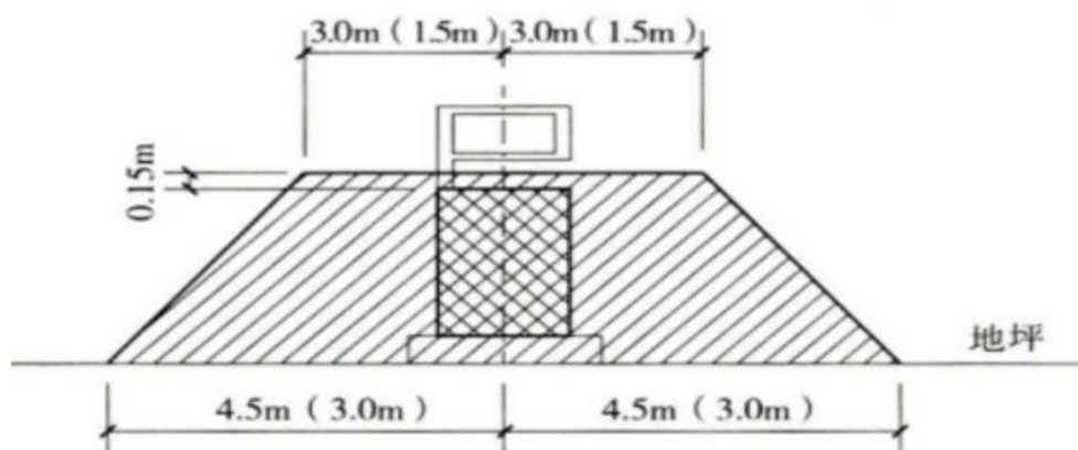
图 1 汽油加油机的爆炸危险区域划分 1区： 2区
